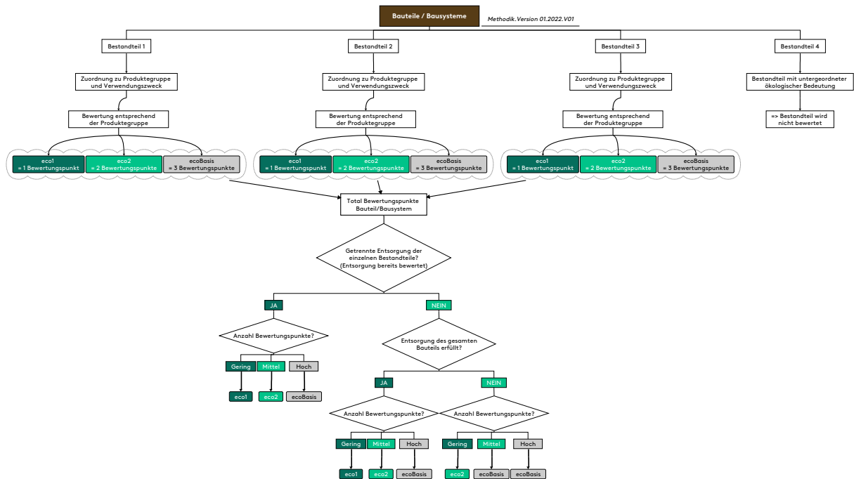
Bild 6: Bewertung von Bauteilen und Bausystemen
