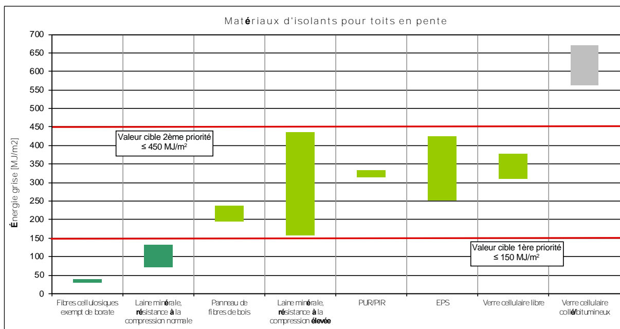
Figure 5: Énergie grise de différents types d'isolants pour toits en pente et valeurs cibles
