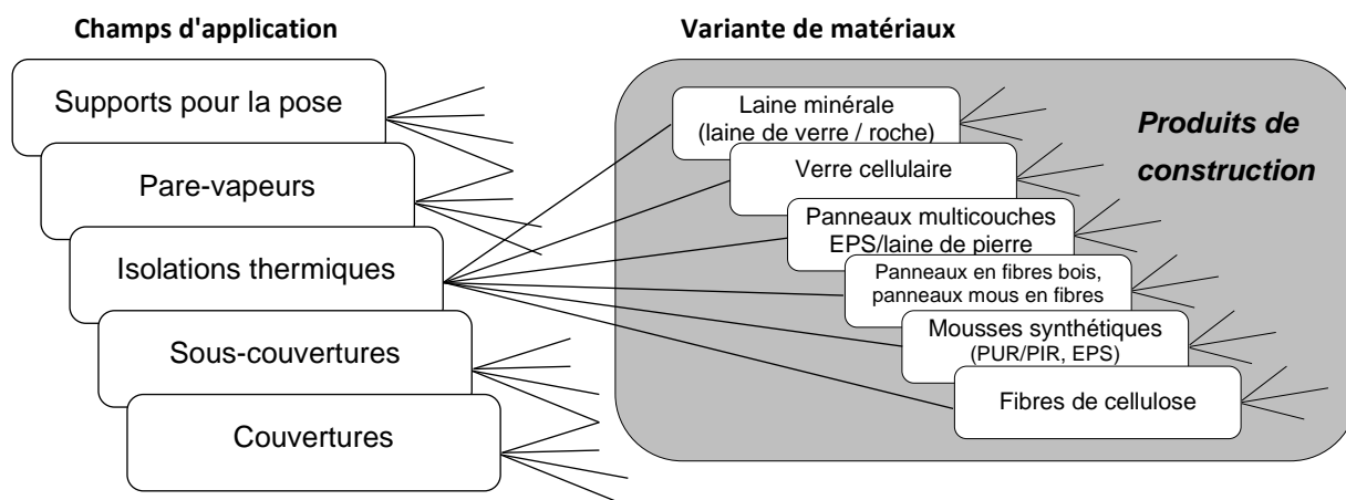
Figure 4: Les champs d'application les plus importants pour l'ensemble des couches d'un toit en pente.
